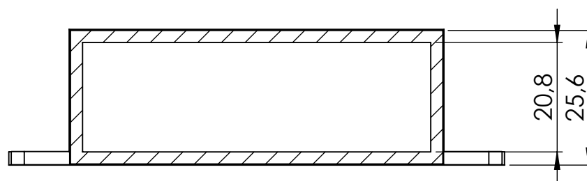
PRZEKRÓJ A-A
