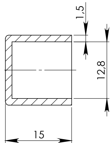
PRZEKRÓJ B-B
